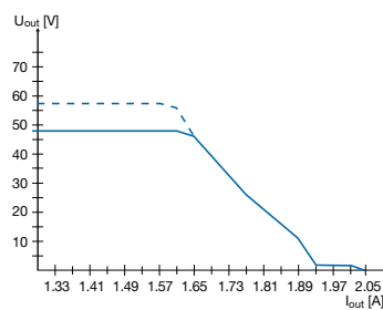
CP-E 48/1.25
