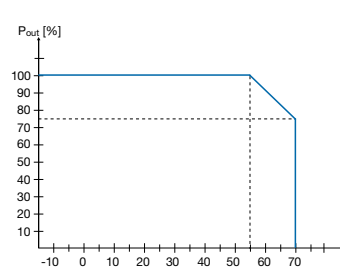
CP-D 24/2.5
