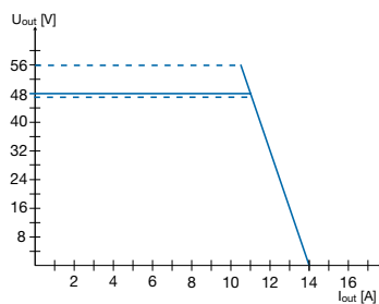
CP-E 48/10.0
