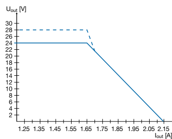
CP-E 24/1.25
