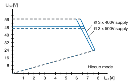
CP-T 48/5.0
