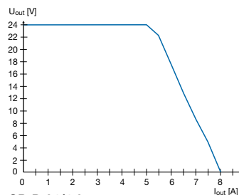
CP-D 24/4.2
