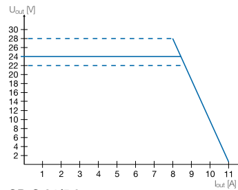
CP-C 24/5.0
