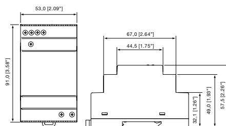
CP-D 12/2.1, CP-D 24/1.3
