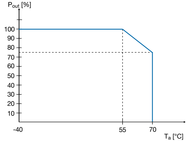
CP-E 24/20.0, CP-E 48/10.0
