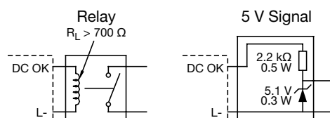
CP-E 24/1.25, CP-E 24/2.5
