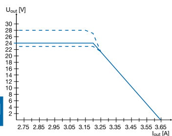
CP-E 24/2.5
