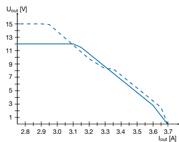
CP-E 12/2.5
