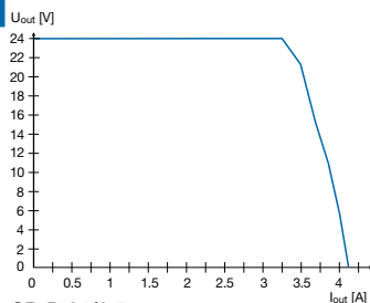
CP-D 24/2.5
