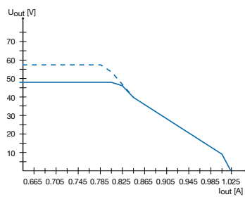
CP-E 48/0.62
