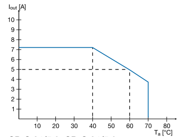
CP-S 24/5.0, CP-C 24/5.0
