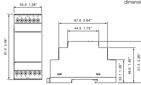
CP-D RU
