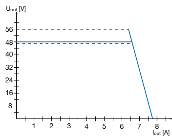
CP-E 48/5.0
