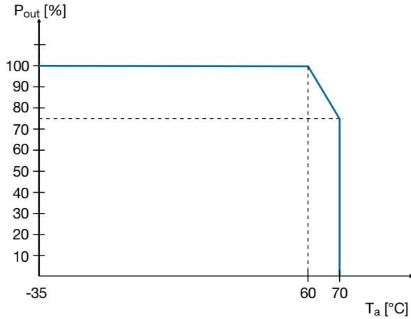
CP-E 12/10.0, CP-E 24/5.0
